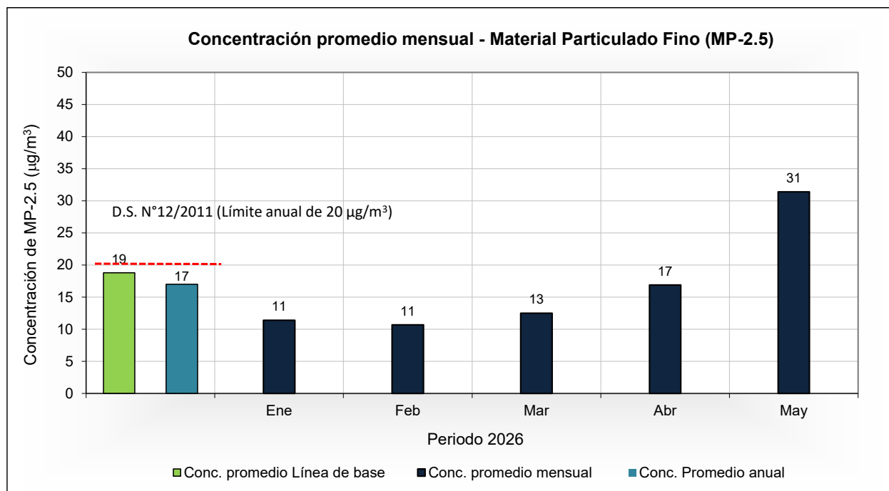
Figura 5 - Concentración promedio mensual de MP-2.5, enero - mayo 2026
