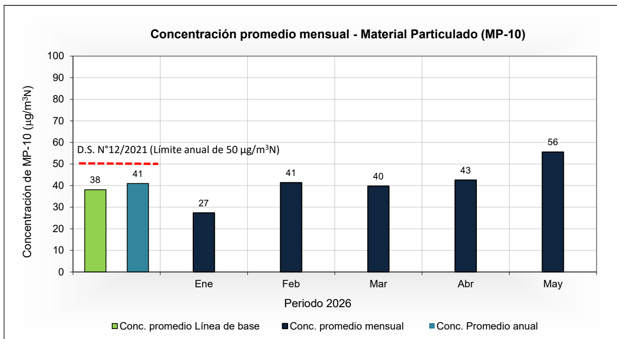
Figura 3 - Concentración promedio mensual de MP-10, periodo enero - mayo 2026
