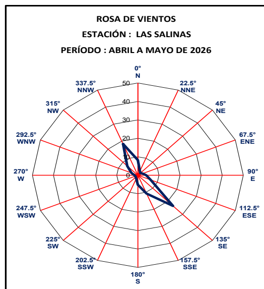
Figura 9 - Rosa de vientos abr-may 2026
