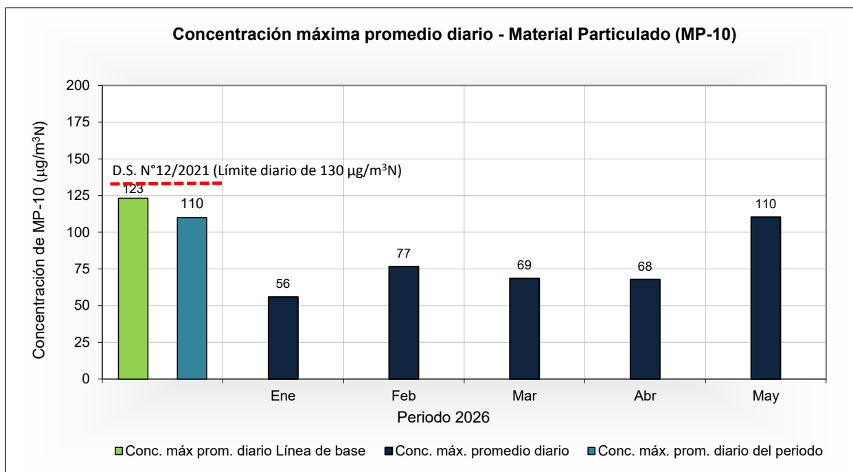
Figura 4 - Concentración máxima promedio diario mensual de MP-10, periodo enero - mayo 2026
