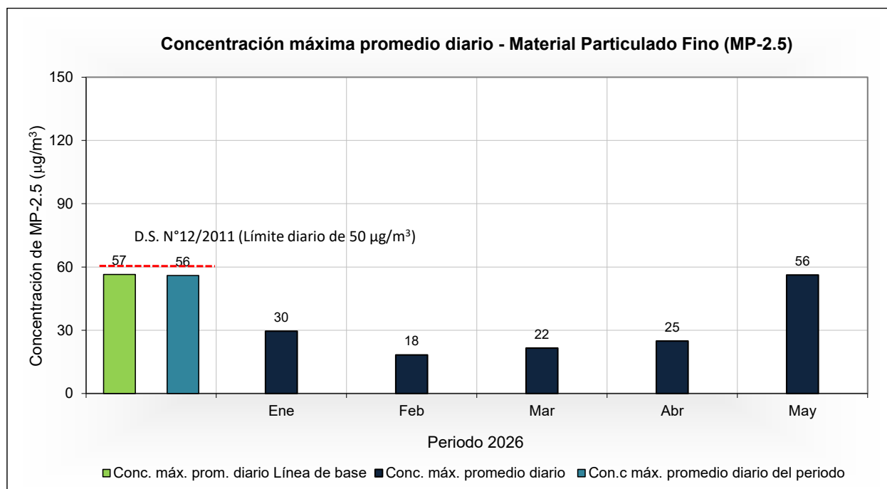
Figura 6 - Concentración máxima promedio diario mensual de MP-2.5, enero - mayo 2026
