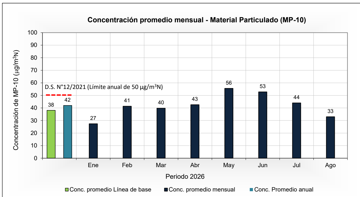
Figura 4 - Concentración promedio mensual de MP-10, periodo enero - agosto 2026
