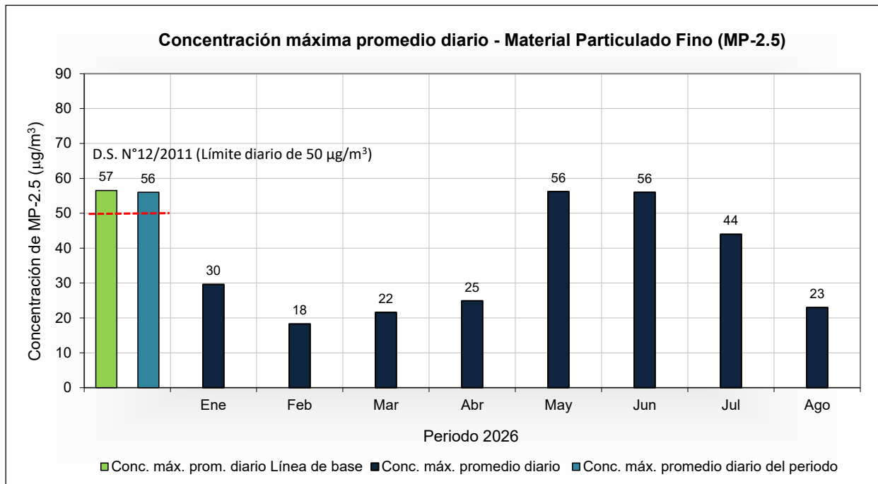
Figura 7 - Concentración máxima promedio diario mensual de MP-2.5, enero - agosto 2026
