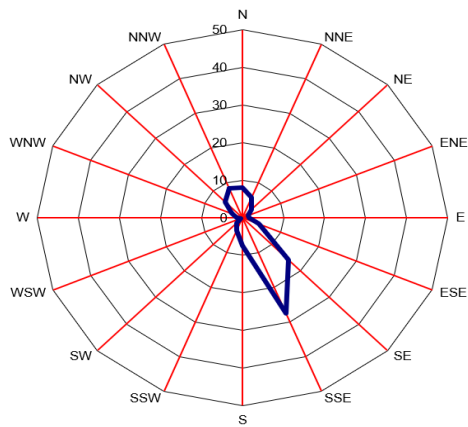
ACUMULADA MENSUAL ESTACIÓN LAS SALINAS AGOSTO DE 2026
