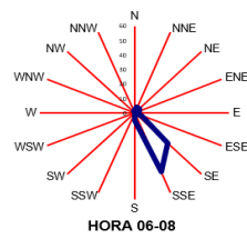
ROSA DE VIENTOS ESTACIÓN LAS SALINAS AGOSTO DE 2026
