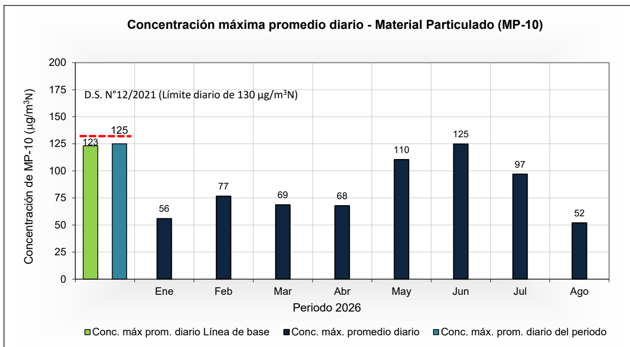
Figura 5 - Concentración máxima promedio diario mensual de MP-10, periodo enero - agosto 2026
