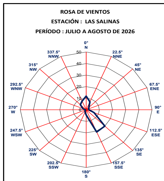
Figura 11 - Rosa de vientos jul-ago 2026
