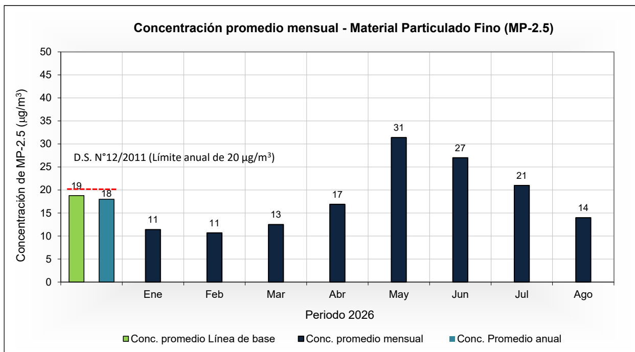
Figura 6 - Concentración promedio mensual de MP-2.5, enero - agosto 2026
