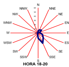
ACUMULADA MENSUAL ESTACIÓN LAS SALINAS AGOSTO DE 2026
